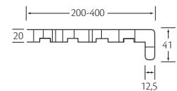
vensterbank 250 mm 2 x 6 m 1 art. nr.: 0762
